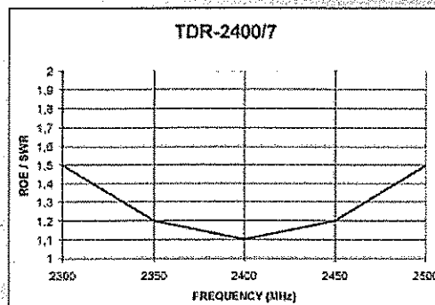
DIAGRAMA DE SWR/ R.O.E.
